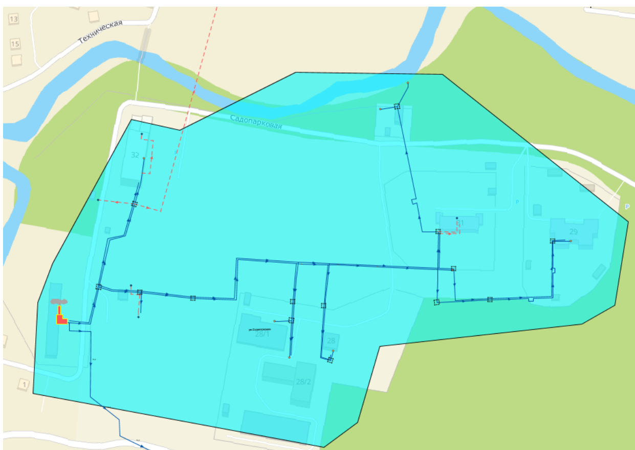
Рисунок 1.21 – Зона действия котельной №32
