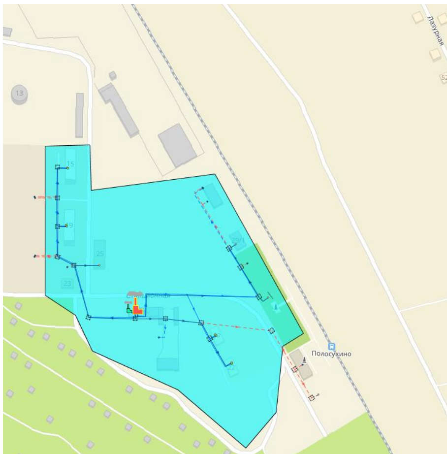
Рисунок 1.34 – Зона действия котельной Полосухинская
