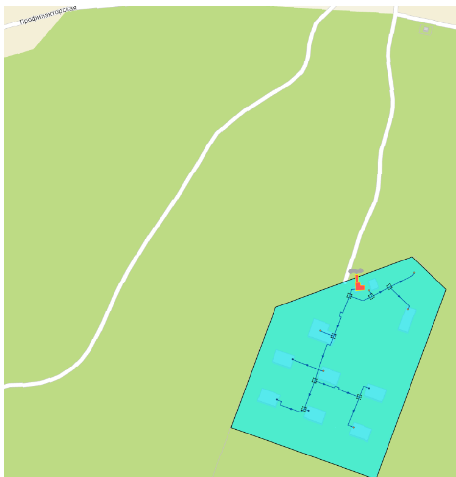
Рисунок 1.31 – Зона действия котельной интернат №66
